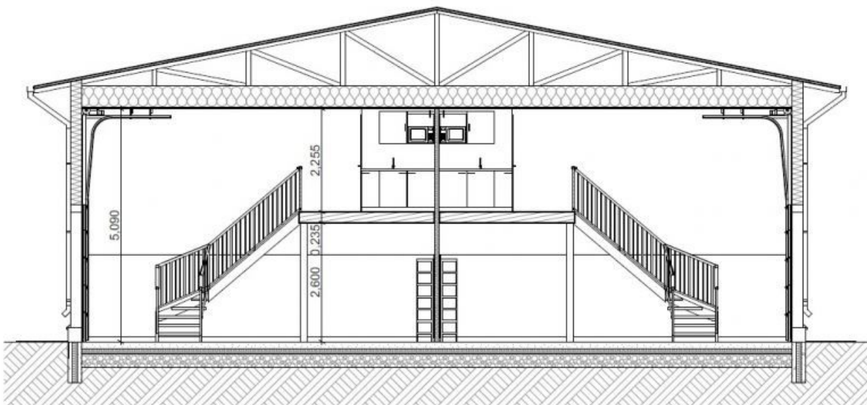
A Leikkaus 1:100
