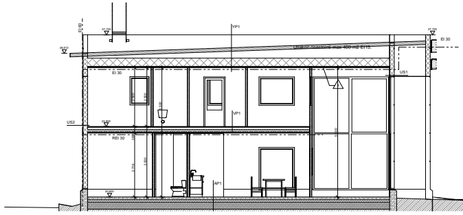
LEIKKAUS A1
