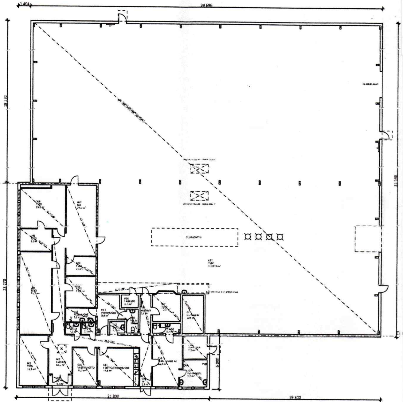
POHJAPIIRROS 1. KRS, 1:100
